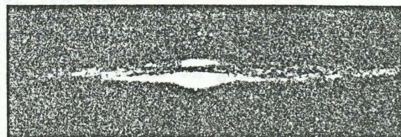
Galaxy in Coma Berenices (NGC 4565)
